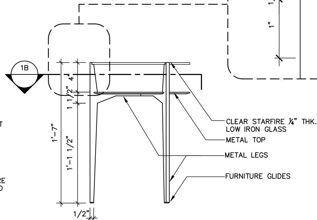
1D ELEVATION SCALE: 1 1/2" = 1'-0"
