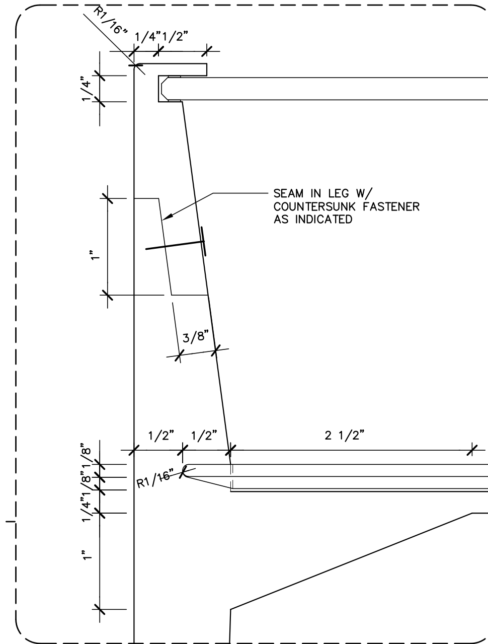
1C SIDE ELEVATION SCALE: 1 1/2" = 1'-0"
