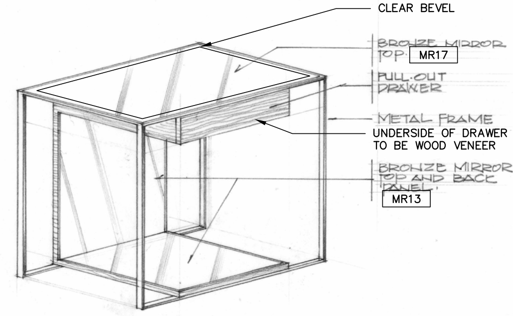
1D AXONOMETRIC SCALE: 1 1/2" = 1'-0"
