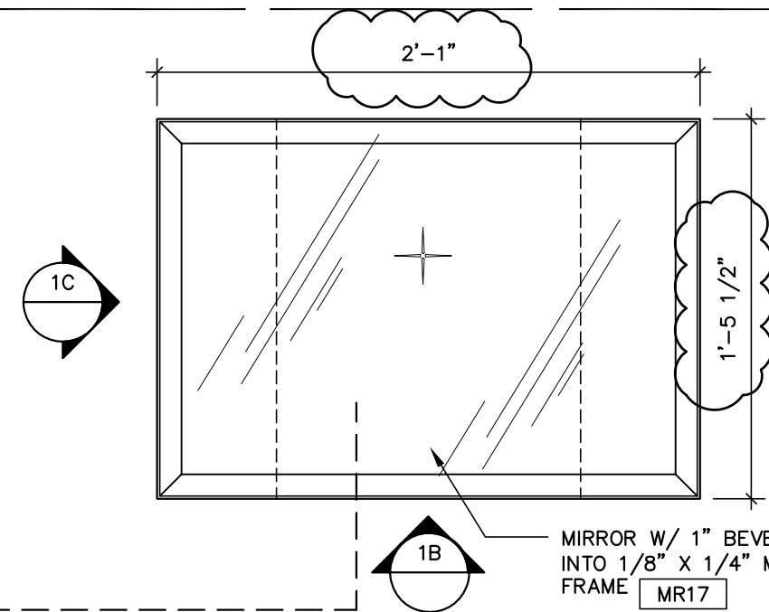
1A PLAN SCALE: 1 1/2" = 1'-0"
