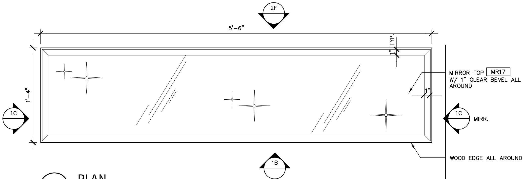
1A PLAN SCALE: 1 1/2"=1'-0"
